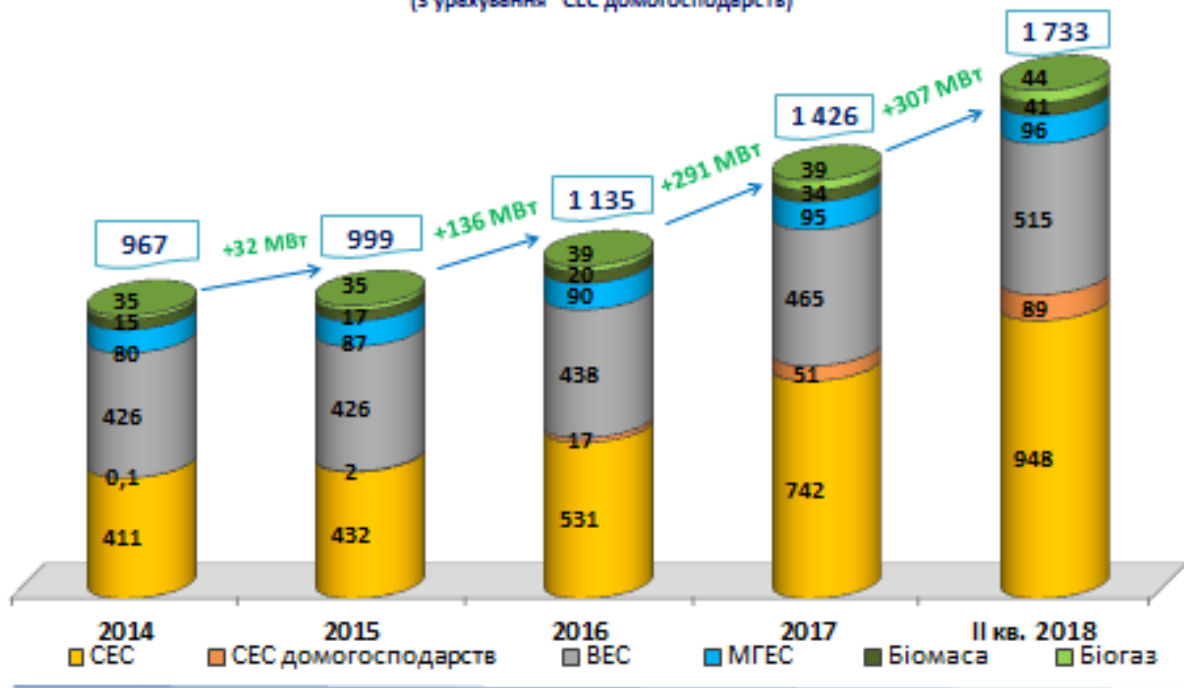
Встановлена потужність об'єктів відновлюваної електроенергетики, що працюють за «зеленим» тарифом, МВт (з урахування СЕС домогосподарств)
